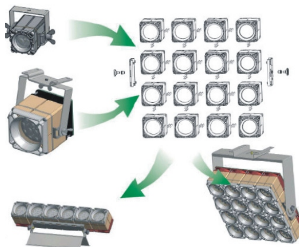
Schemat budowy opraw modułowych
